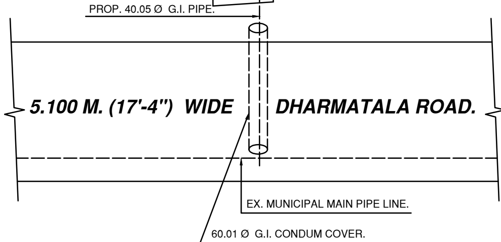
SITE PLAN.
